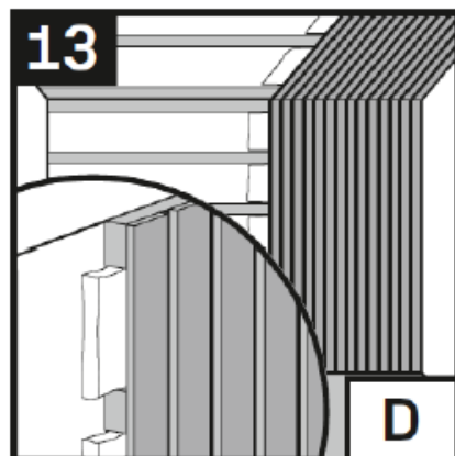
Vissage à la sous-structure + isolation Classe d'absorption A
