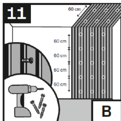
Raccordement direct par vis tous les 60 cm Classe d'absorption D
