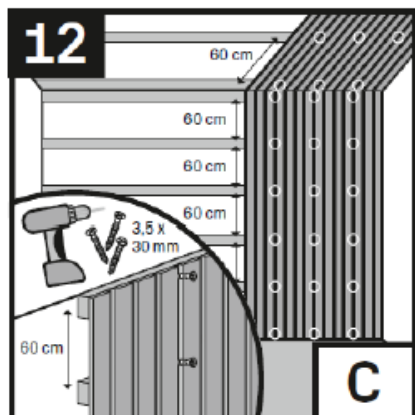
Vissage à la sous-structure Classe d'absorption B (100mm) Classe d'absorption C (60mm)
